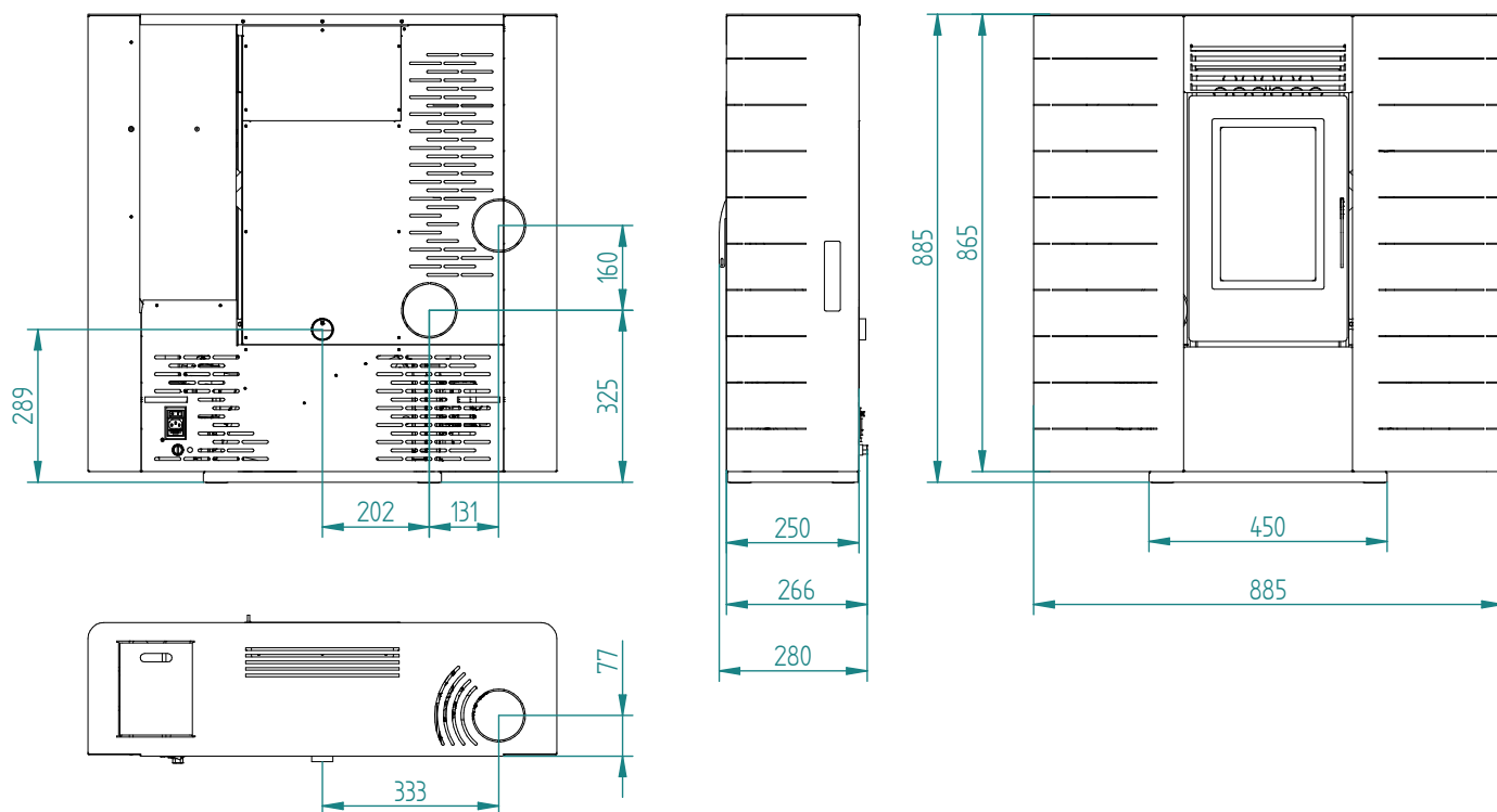
Fig.4: dimensionamento modello 60
