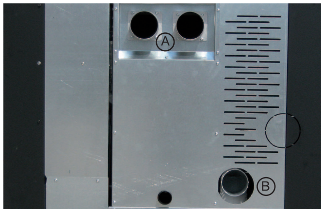
A. Canalizzazione orizzontale ove presente B. Estrazione fumi
