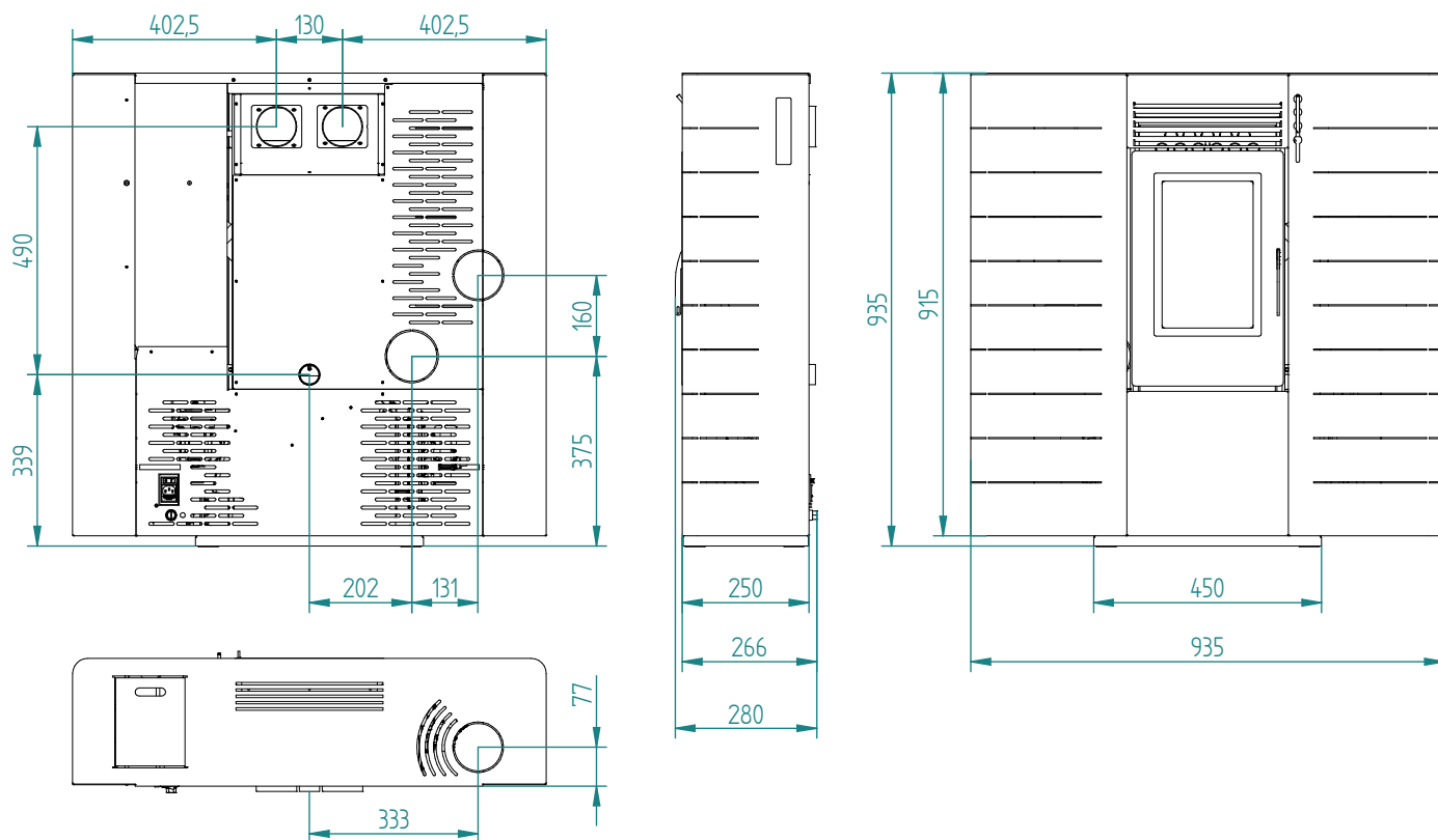
Fig.5: dimensionamento modello 90
