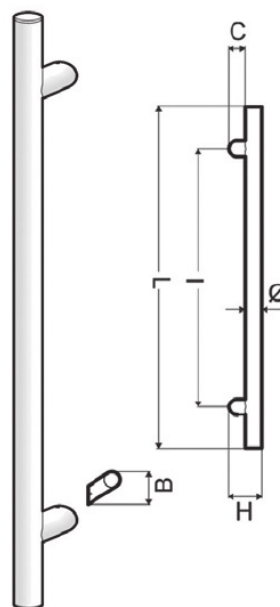
SUPPORTI INCLINATI
